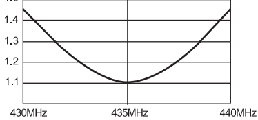
V.SWR chart (X-200N)
